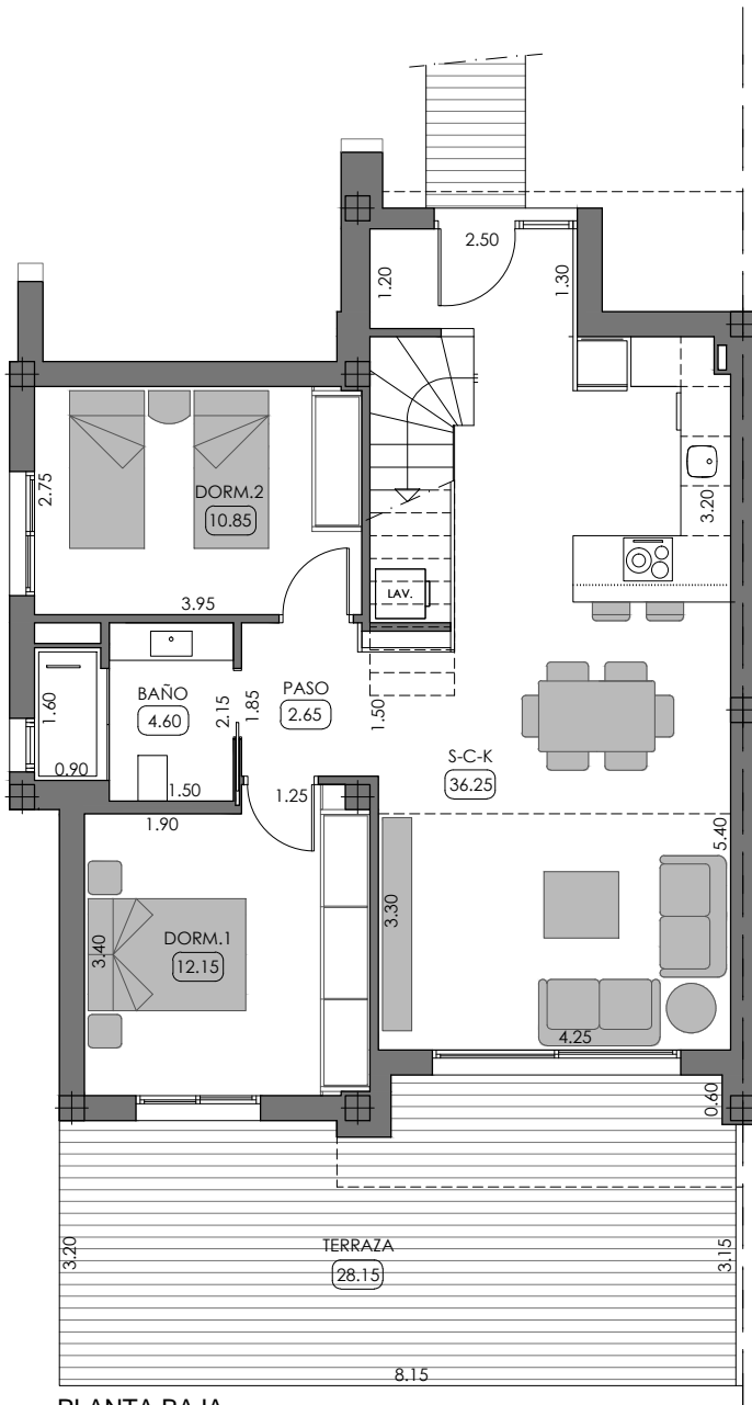
PLANTA BAJA
