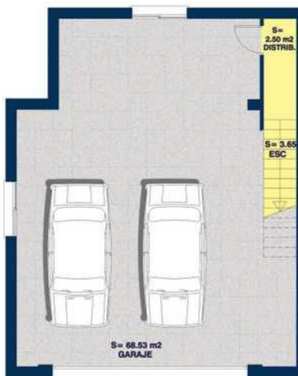
PLANTA SOTANO
